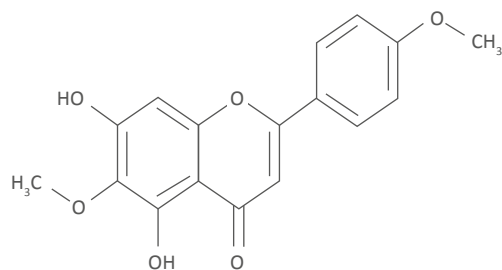
D. 5,7- dihidroxi-4',6 -dimetoxiflavona
