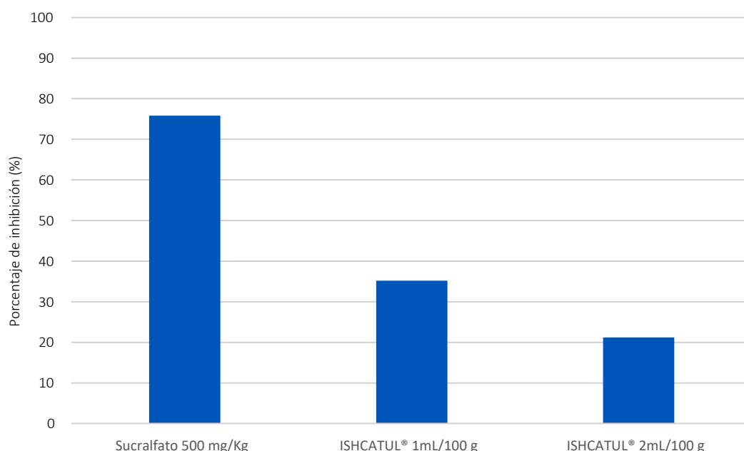
Gráfico N°02. Porcentajes de inhibición de formación de úlcera gástrica por grupos de estudio en comparación al control negativo.
