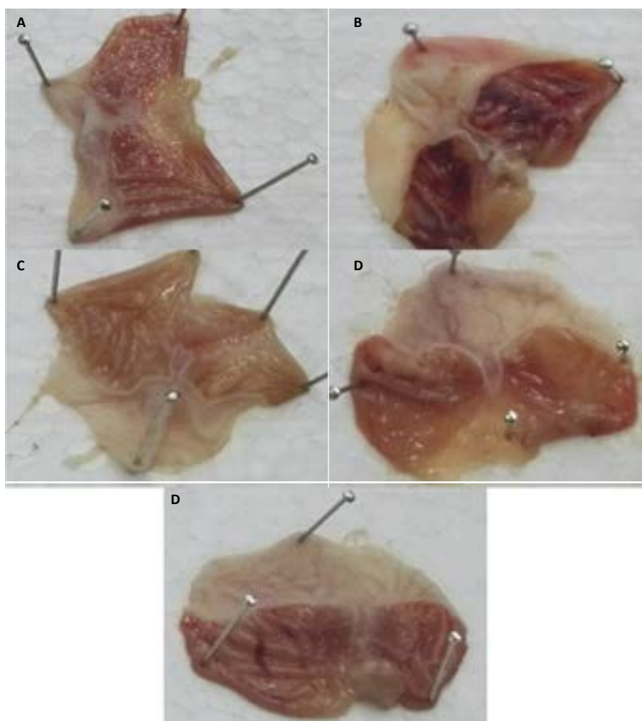
Gráfico N°01. Observación directa de estómagos de modelo experimental por grupo de estudio. A) Blanco; B) Control negativo; C) Control positivo; D) Cocimiento de ISHCATUL® (1mL./100 g); D) Infusión de ISHCATUL® (2mL./100 g).
